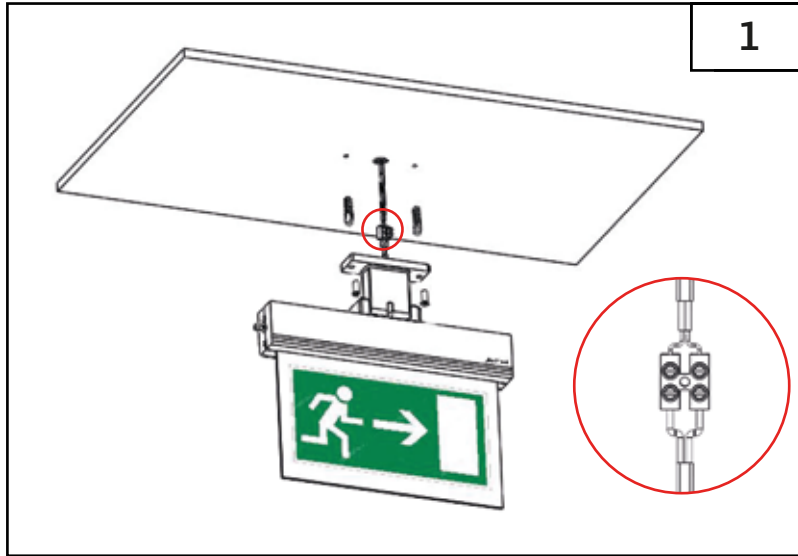
1.2 Ölçülere uygun bağlantı delikleri delinir. Ürün kasası civatalarla tavana monte edilir. 1.2 Connection holes are drilled in accordance with the dimensions. The product casing is mounted to the ceiling with bolts.
