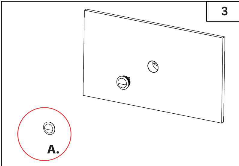
3.1 Armatür kasaya monte edilir. 3.1 The product is mounted. A. Armatürün yanlarından duvar boşluğu gözükmecek şekilde eksentreyiniz. A. Cented the sides of the to reach the luminaires.
