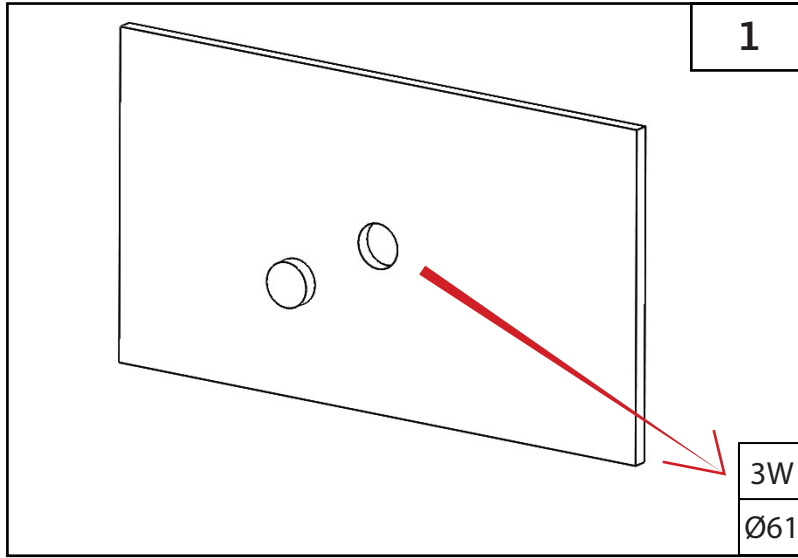
1.1 Ölçülere uygun bağlantı delikleri delinir. 1.1 Connection holes are drilled in accordance with the dimensions.
